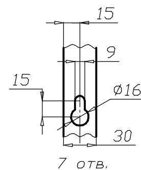
В (увел.)
