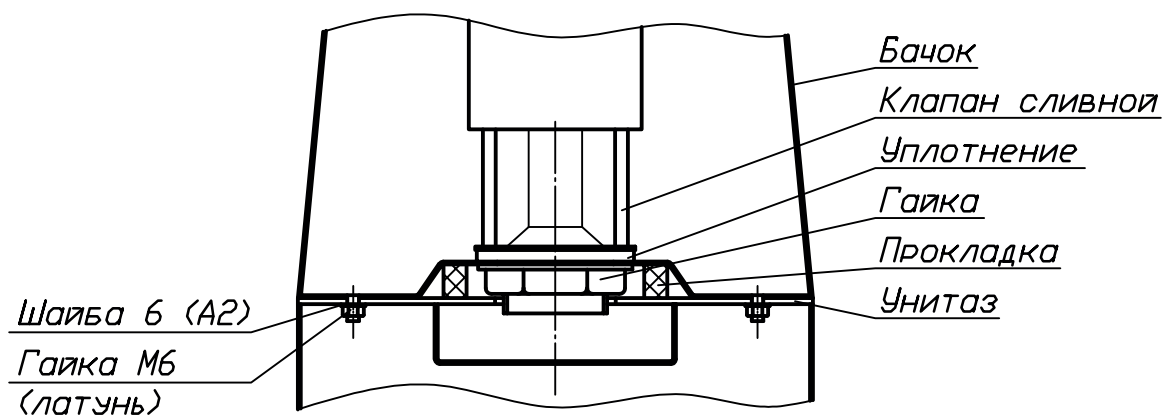
Схема установки бачка
