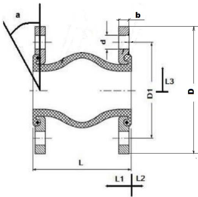
Рисунок 2 - Размеры
