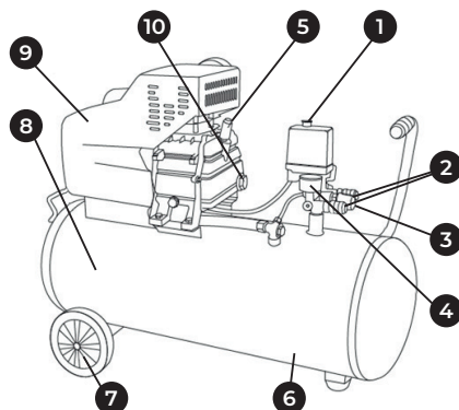
Рис. 1.1 (компрессор с прямой передачей)
