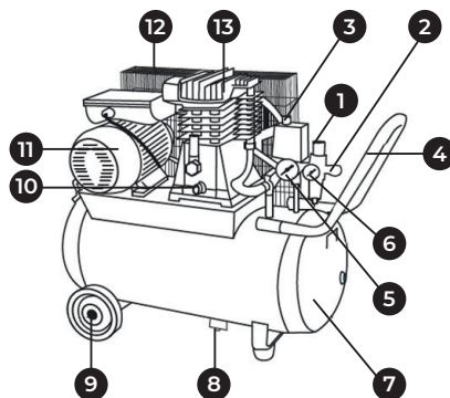
Рис. 1.2 (компрессор с ременной передачей)
