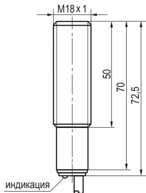
Габаритный чертеж
