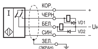
Схема подключения индуктивной нагрузки
