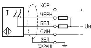
Схема подключения активной нагрузки
