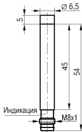
Габаритный чертеж
