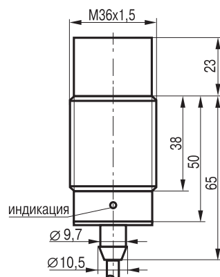
Габаритный чертеж
