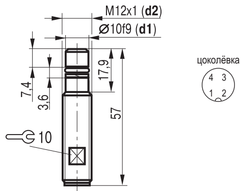
Схема монтажа
