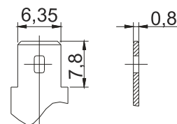
Клемма F2
