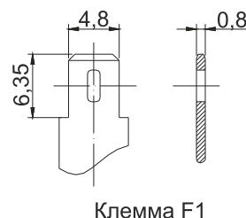
Клемма F1
