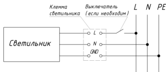
Рисунок 2 – Подключение светильника к сети ~220В.
