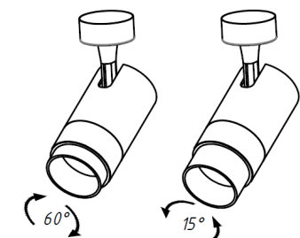
Рисунок 4 – Регулировка угла рассеивания.
