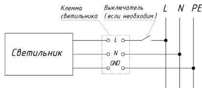
Рисунок 3. Схема подключения светильника.
