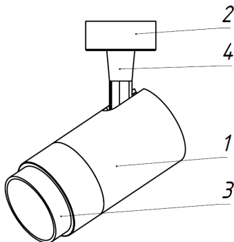
Рисунок 2. Конструкция светильника.
