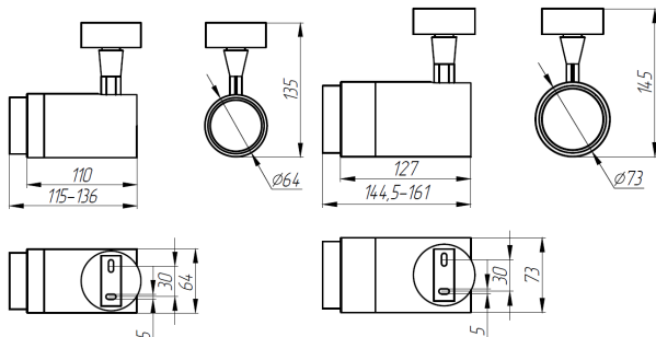
Рисунок 1. Габаритный чертеж: а) Track Classic Zoom 10Вт, б) Track Classic Zoom 20Вт.
