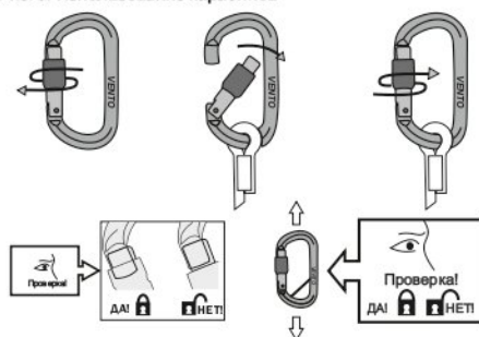
Рис. 3. Использование карабинов
