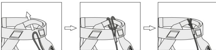
Рис. 5. Крепление усов самостраховки
