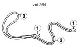
Рис. 1. Внешний вид, состав усов самостраховки
