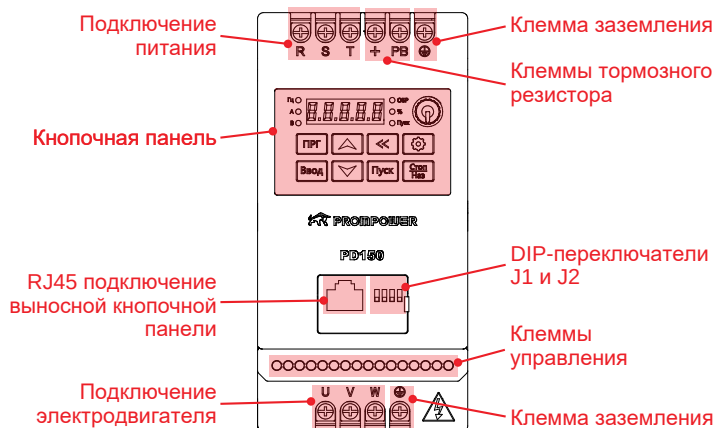
Рисунок 3-1 Расположение клемм преобразователей частоты PD150-A_004B, PD150-A_007B, PD150-A_015B, PD150-A4022B
