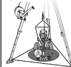
Рис. 17. Пример организации системы канатного доступа
