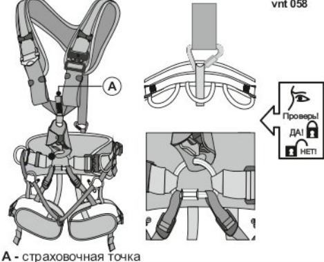
Рис. 2. Компоненты страховочной привязи «Профи Пихта» vnt 058
