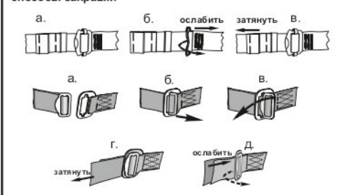
Рис. 9. Соединительно-амортизирующая подсистема
