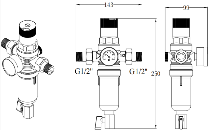
Размеры клапанов (ширина включает размер манометра)
