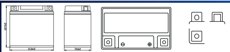
Габариты
