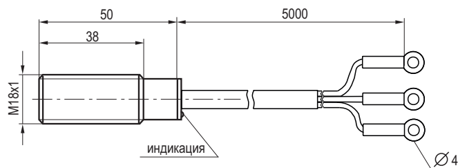
Габаритный чертеж
