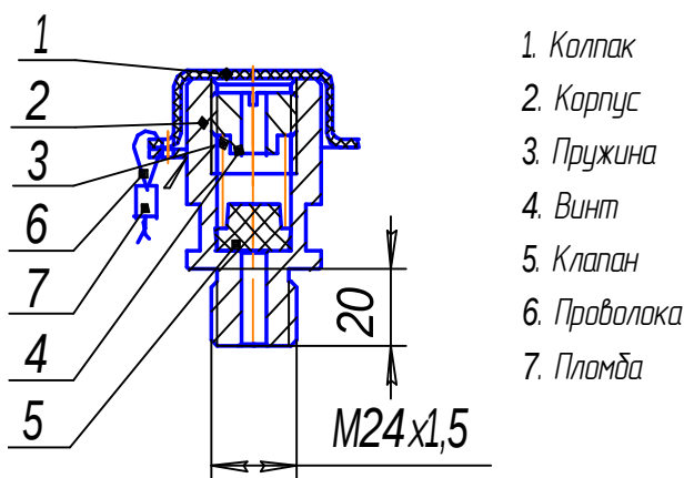
Рис.5 – Предохранительный клапан (отрегулирован на срабатывание при давлении 15 кгс/см 2 )
