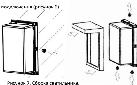
Рисунок 7. Сборка светильника.
