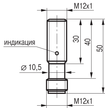
Габаритный чертеж
