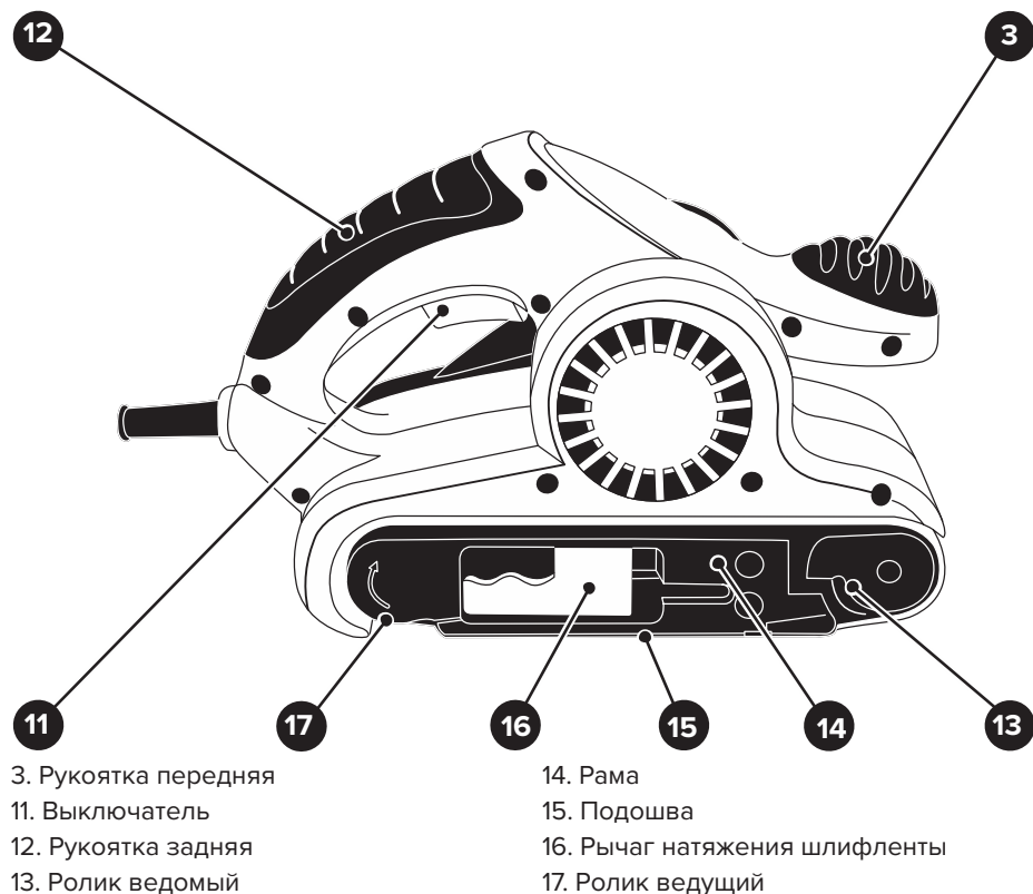
Рисунок 2 — Общий вид шлифмашины
