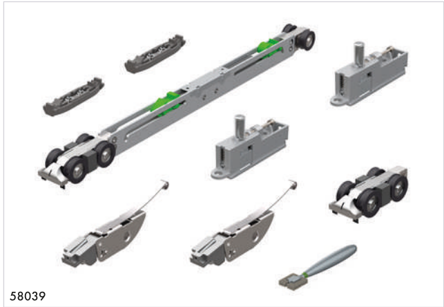
58039 Комплект для раздвижной двери SET3 2 компл.
