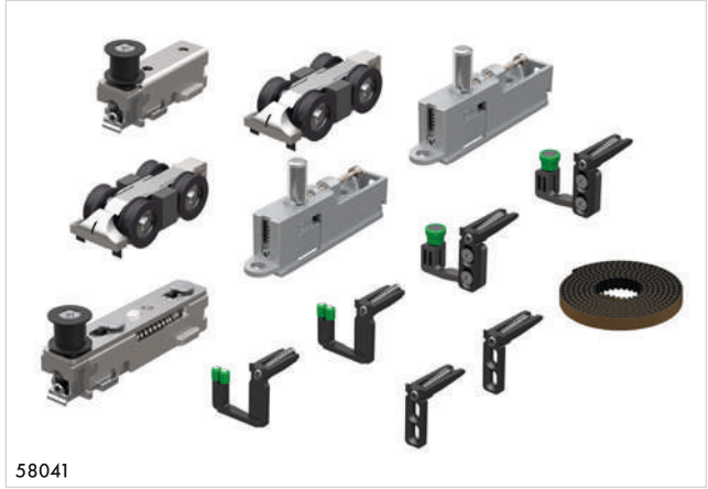
58041 Комплект для телескопического открывания SET5 1 компл.
