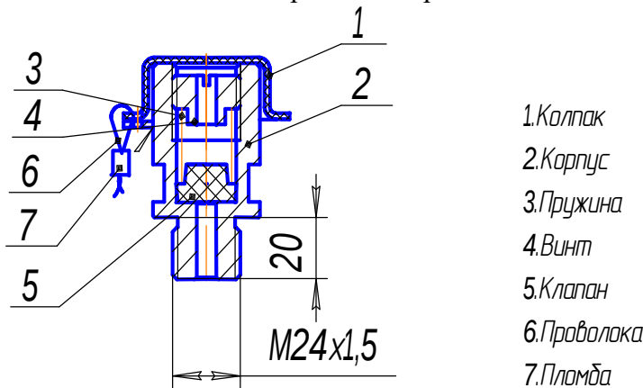
Рис.5 - Предохранительный клапан
