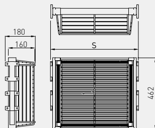
pełny wysuw / full extension / полное выдвижение
