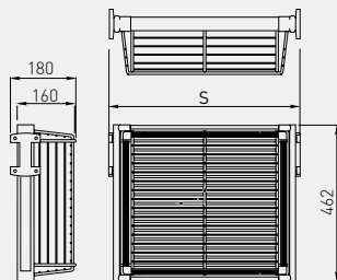
niepełny wysuw / partial extension / неполное выдвижение
