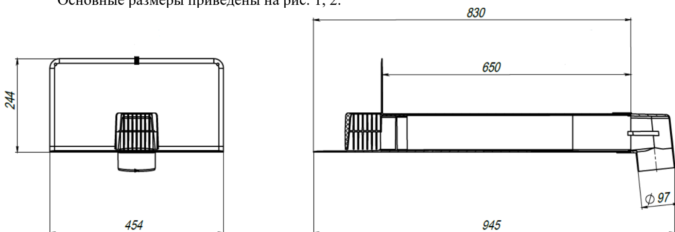
Рис. 1. Парапетная воронка серии VC-PP с листоуловителем и угловым отводом
