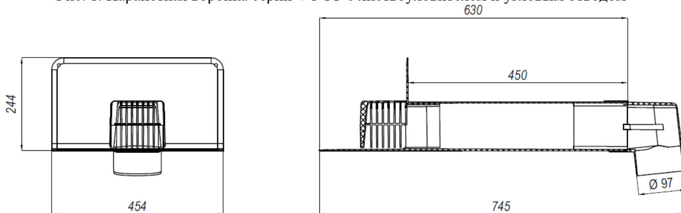
Рис. 1. Парапетная воронка серии VC-PP укороченная с листоуловителем и угловым отводом
