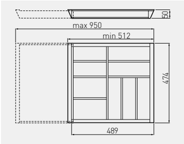
Maksymalny wysuw = 950 mm Maximum extension = 950 mm Максимальное выдвижение = 950 мм
