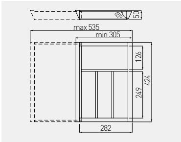
Maksymalny wysuw = 535 mm Maximum extension = 535 mm Максимальное выдвижение = 535 мм
