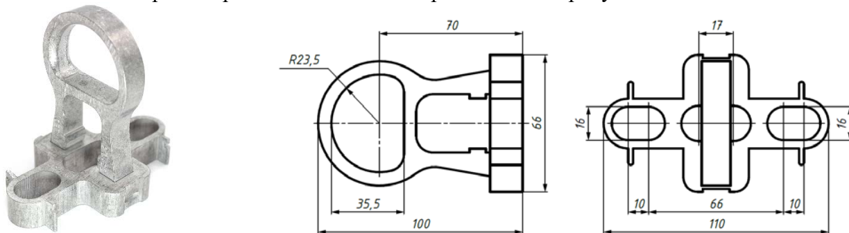
Рис. 1. Внешний вид анкерного кронштейна СА 2000.
