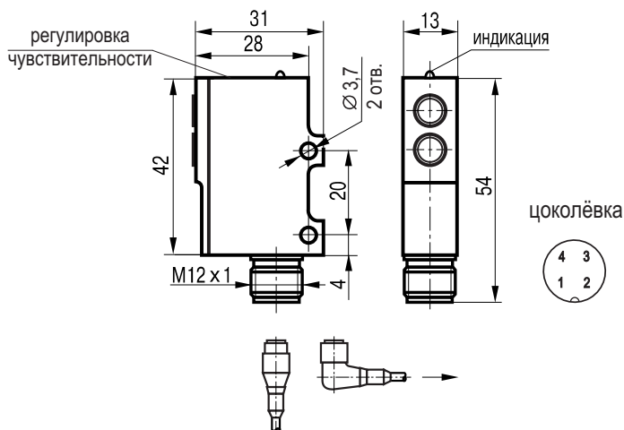
Габаритный чертеж.
