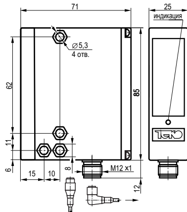
Габаритный чертеж.
