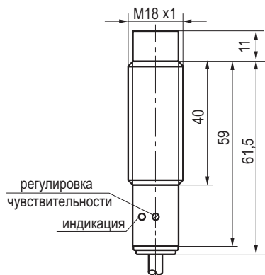
Габаритный чертеж
