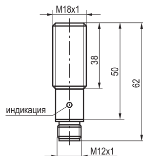
Габаритный чертеж
