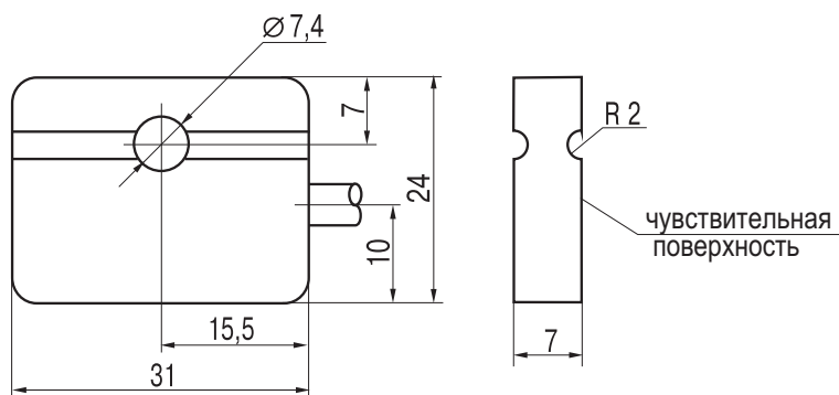
Габаритный чертеж
