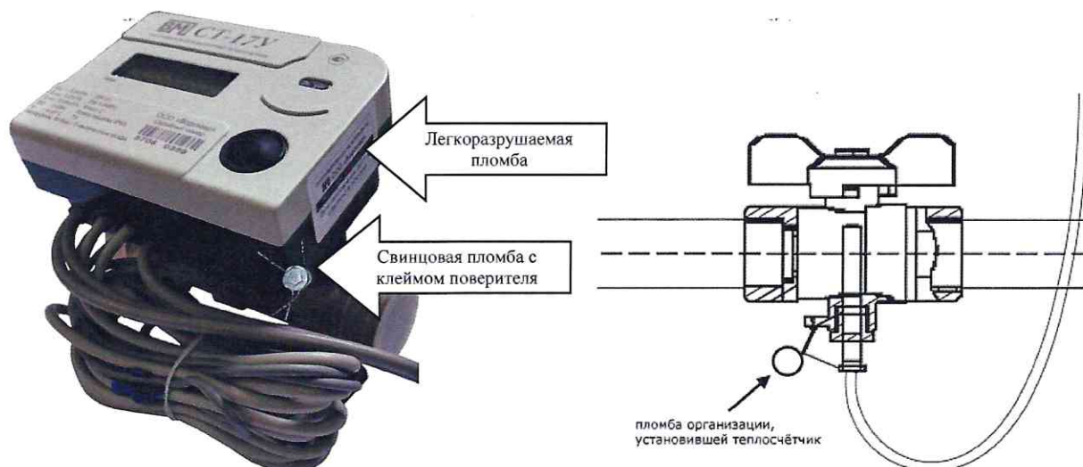
Рисунок 2 – Схема пломбировки теплосчётчиков CT-17Y
