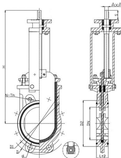
Рисунок 2 - Размеры
