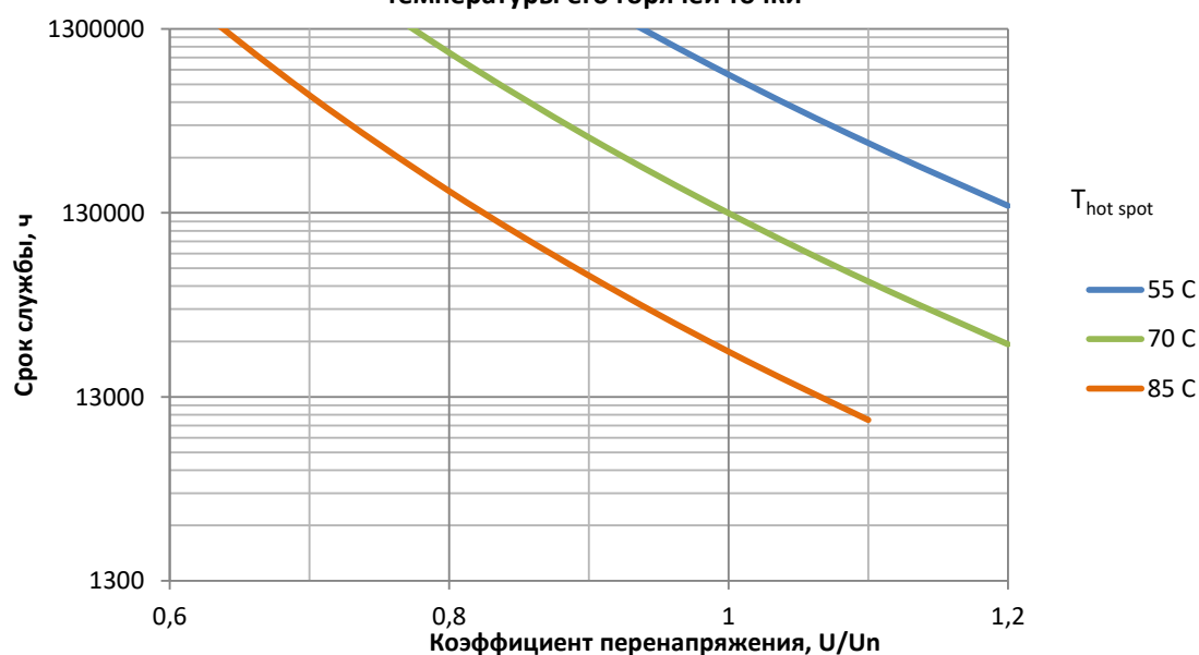
Зависимость ожидаемого срока службы конденсатора от напряжения и температуры его горячей точки
