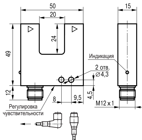
Габаритный чертеж
