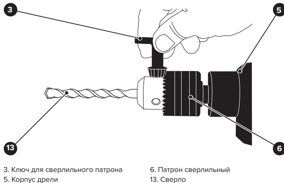
Рисунок 4 — Установка и закрепление сверла в сверлильном патроне
