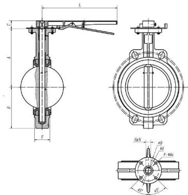
Рисунок 2. Размеры
