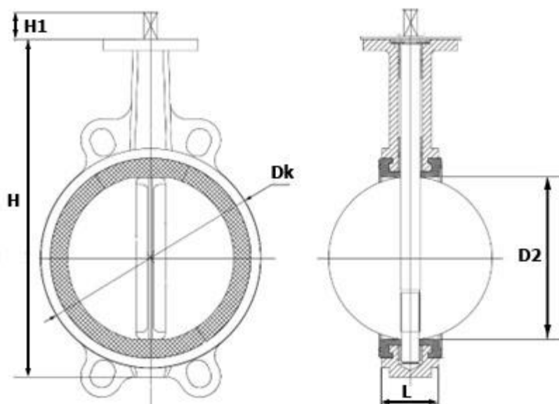
Рисунок 5 – Размеры для DN40 (без рукоятки)
