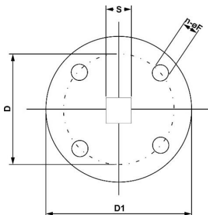
Рисунок 6 – Размеры ISO фланца для DN40 (без рукоятки)
