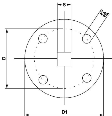
Рисунок 4 – Размеры ISO фланца
