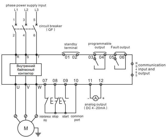
AJR3-3000 схема управления
