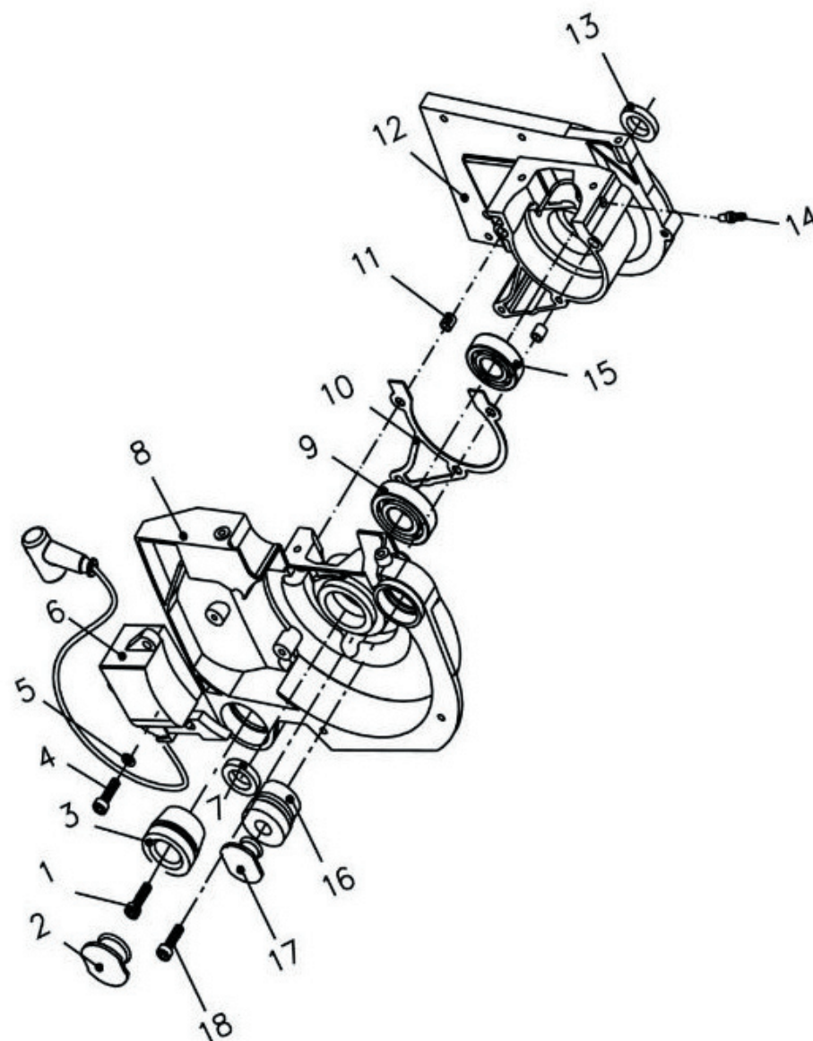
Схема сборки № 9
