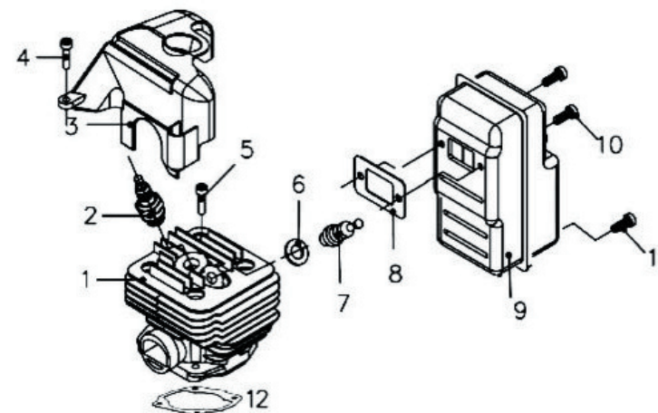
Схема сборки № 7
