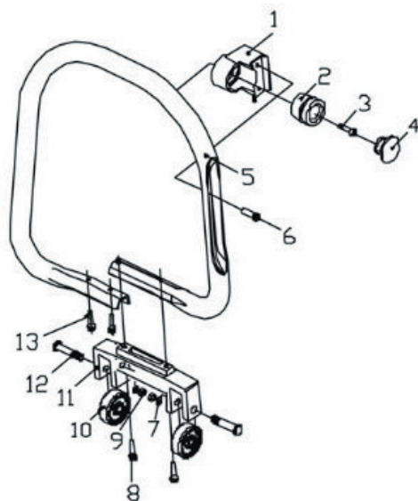
Схема сборки № 1
