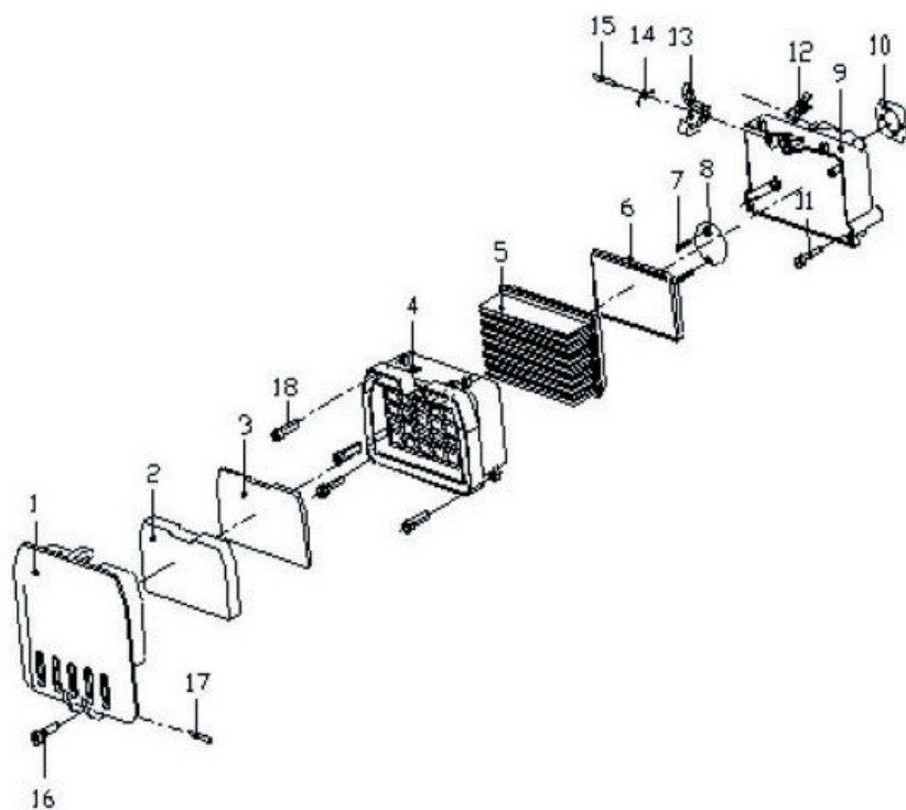
Схема сборки № 3
