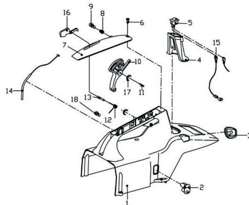
Схема сборки № 4
