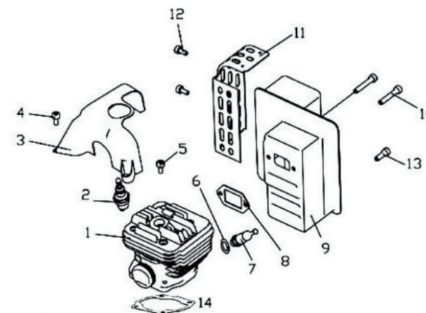
Схема сборки № 6
