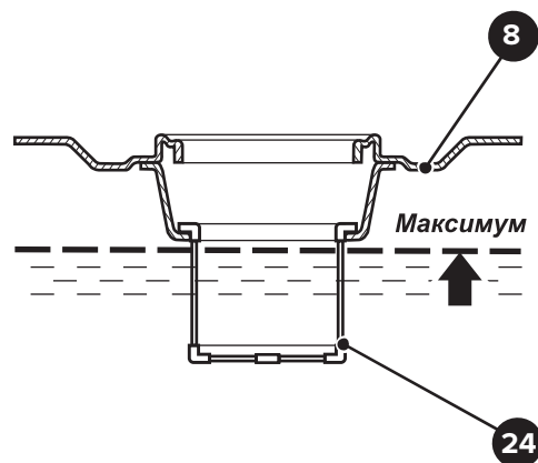
24. Сетчатый фильтр
