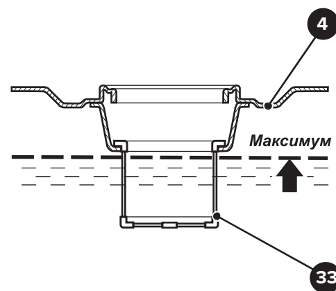
33. Сетчатый фильтр
