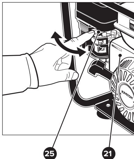
Рисунок 16 — Регулирование частоты вращения двигателя мотопомпы
