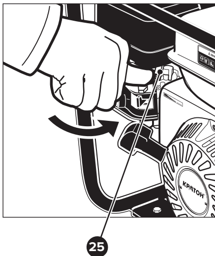
Рисунок 15 — Установка рычага газа в положение «МИН» после запуска двигателя мотопомпы
