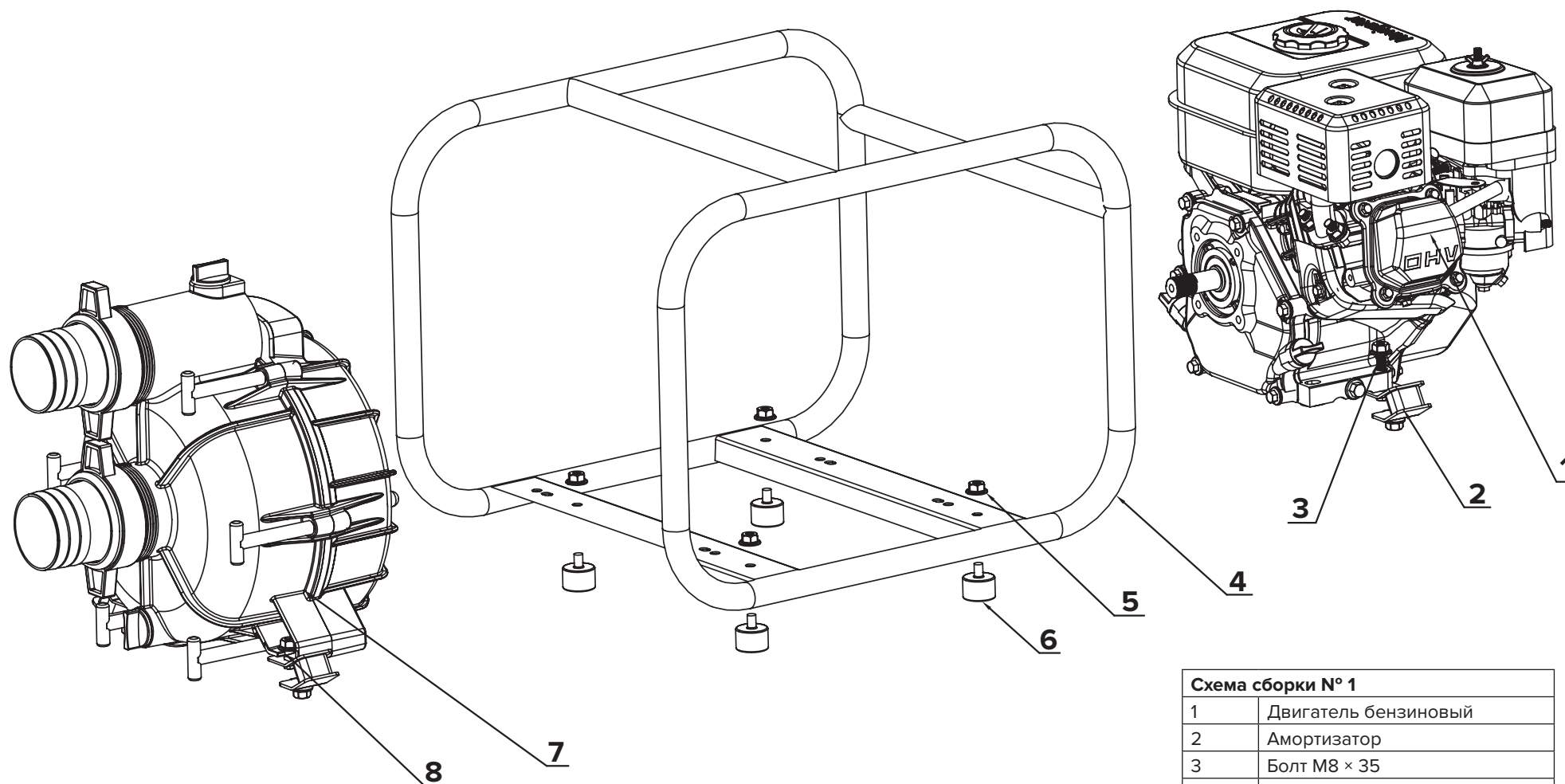
Схема сборки № 1
