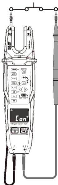
Проверка цепи на обрыв
